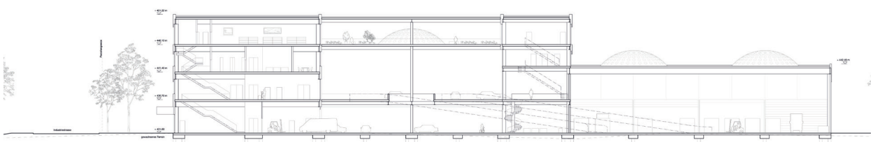
Längsschnitt
