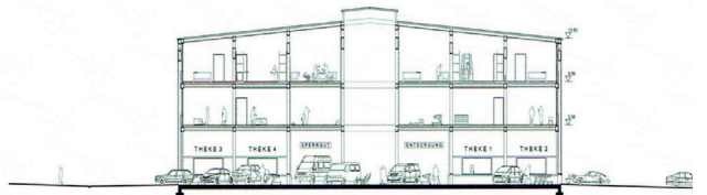
Querschnitt Warenannahme
