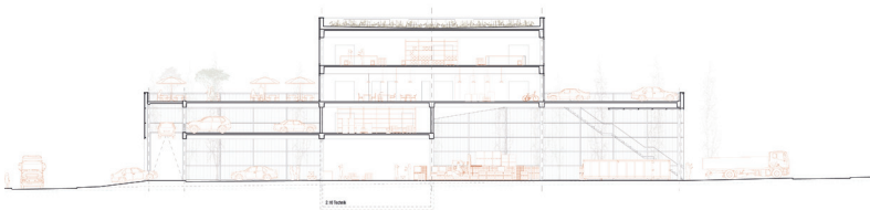
Querschnitt
