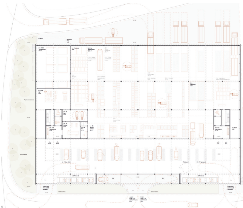
Erdgeschoss
