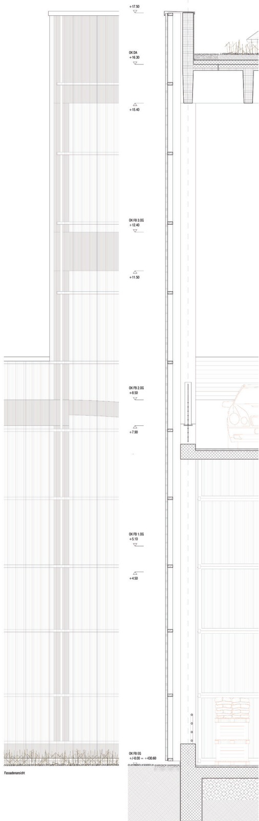
Detailschnitt/-ansicht
