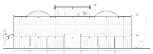
Querschnitt Erschliessung/Parkierung
