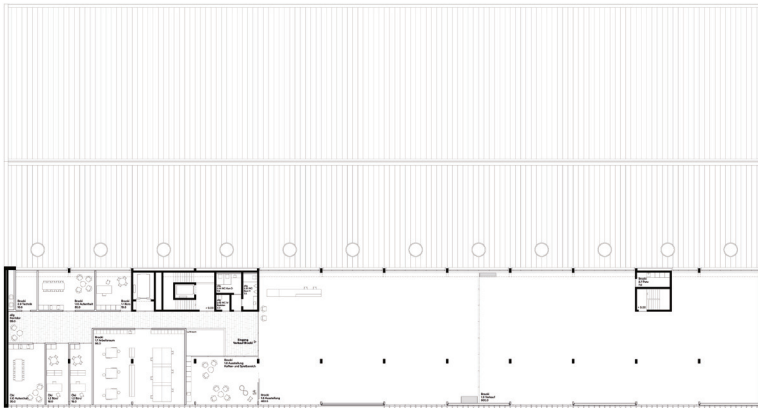
2. Obergeschoss
