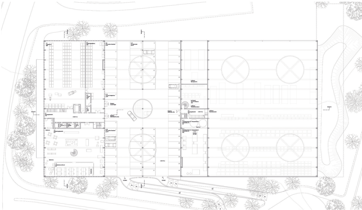
1. Obergeschoss
