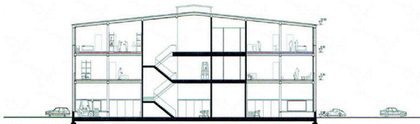
Querschnitt Erschliessung
