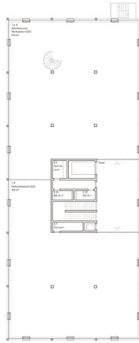
2. Obergeschoss
