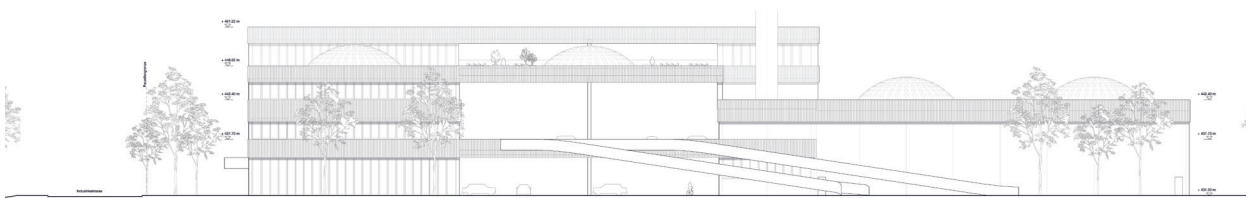
Ansicht Süd
