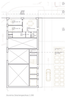
Zwischengeschoss
