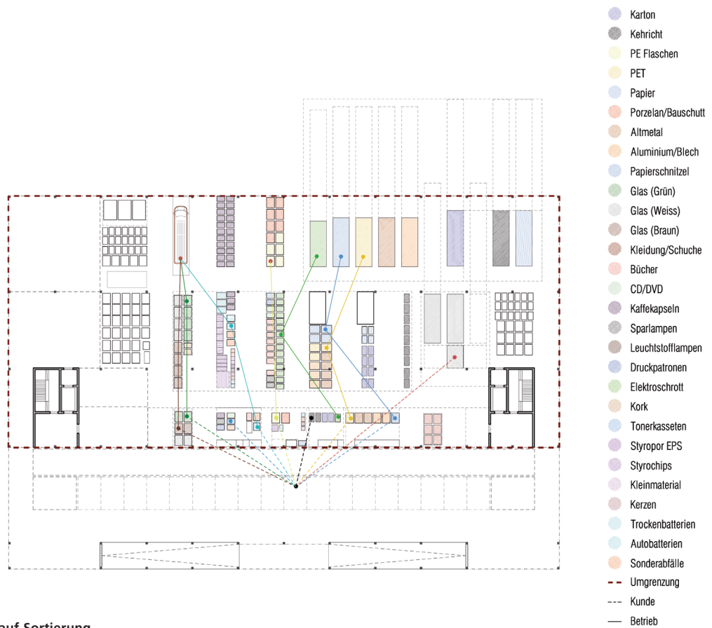
Betriebsablauf Sortierung
