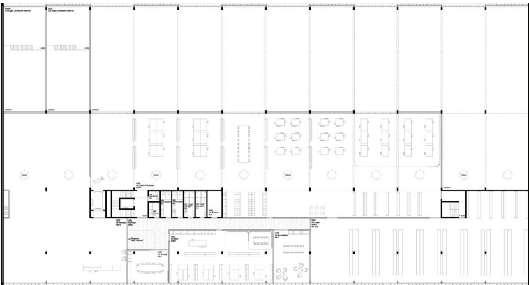
1. Obergeschoss
