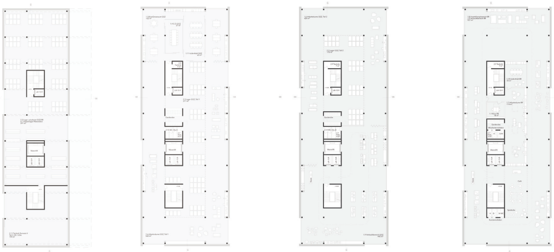
1. bis 4. Obergeschoss
