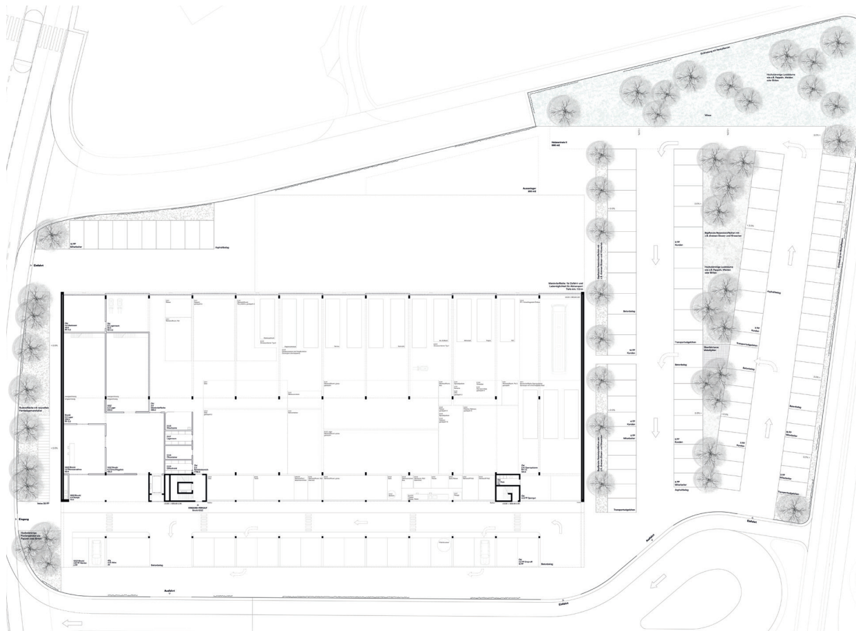
Erdgeschoss
