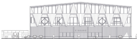
Ansicht West
