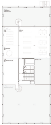
Galerie 1. Obergeschoss
