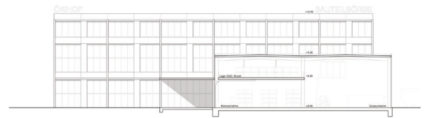
Ansicht Ost
