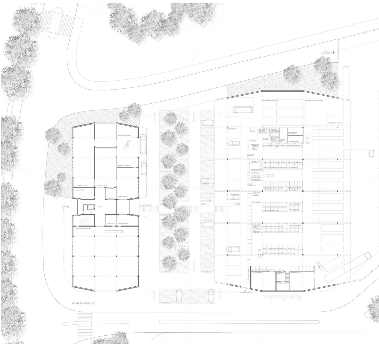
Erdgeschoss
