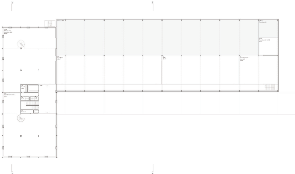
1. Obergeschoss
