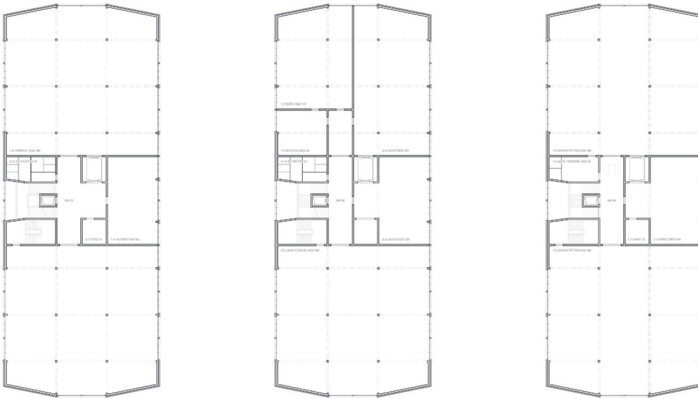
1. – 3. Obergeschoss
