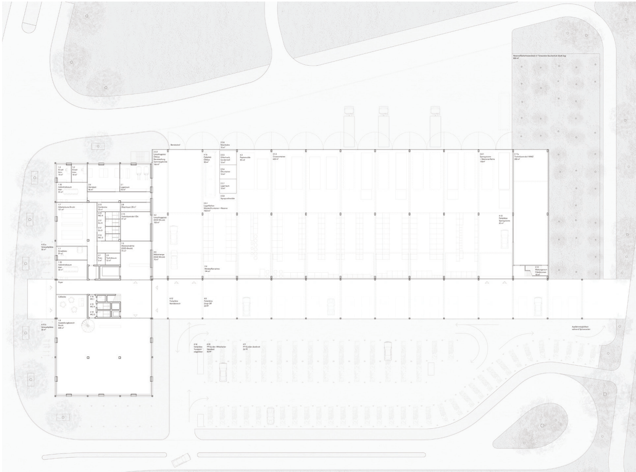
Erdgeschoss
