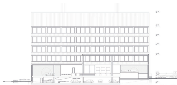
Ansicht Südost
