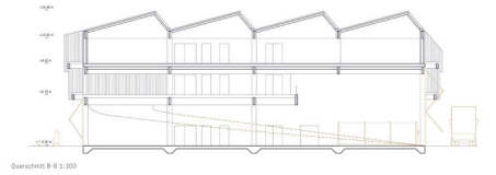
Querschnitt B-B 1:200
