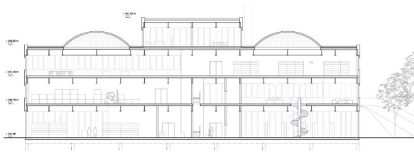
Querschnitt Brockenhaus/GGZ
