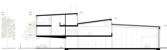
Querschnitt
